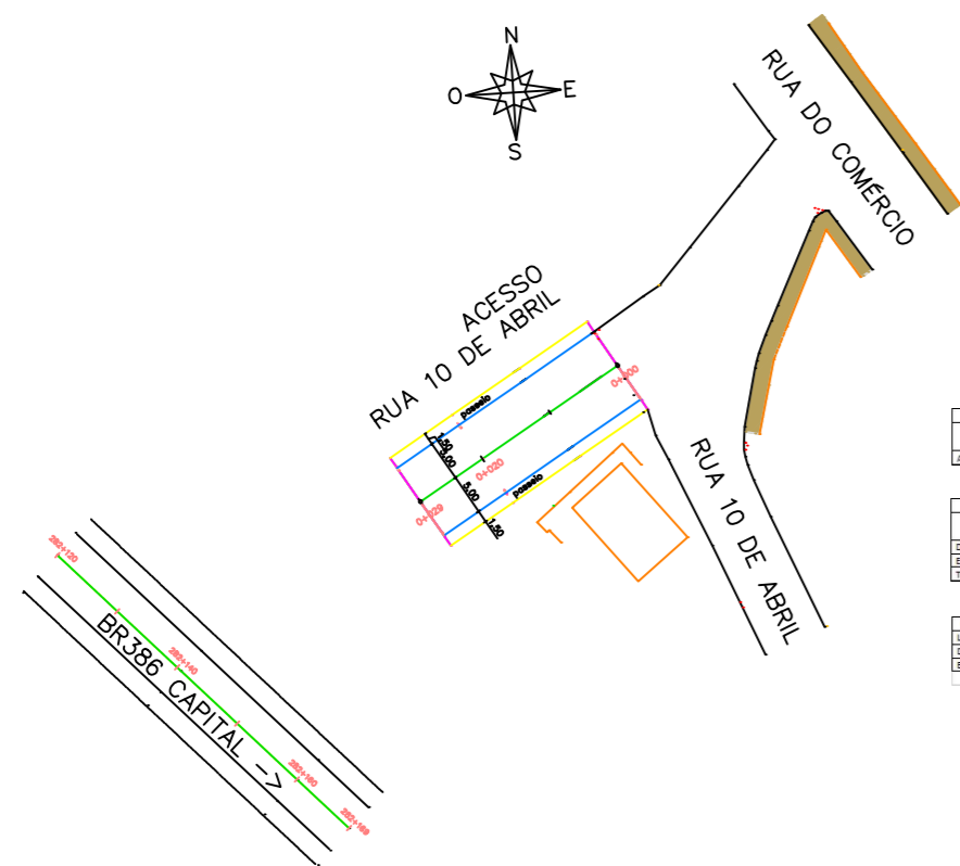
PROJETO GEOMÉTRICO
