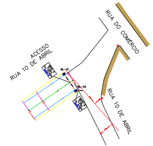
PROJETO DRENAGEM
