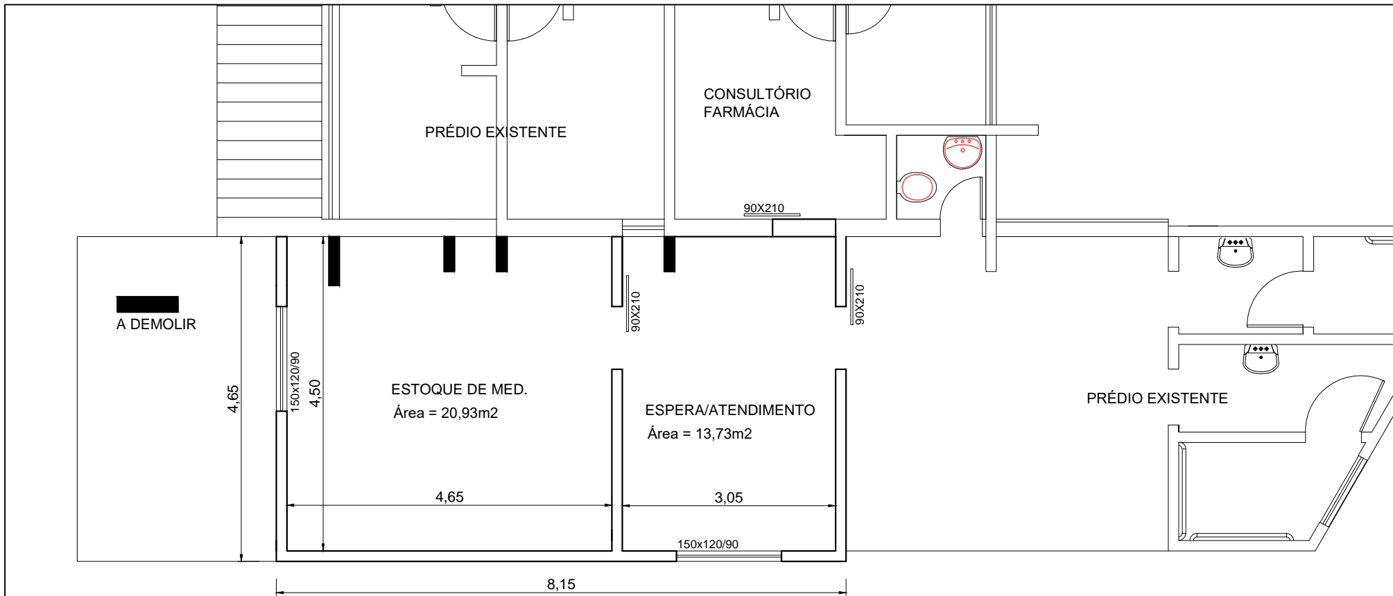
PLANTA BAIXA Área = 37,89m 2
