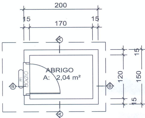
PLANTA BAIXA
